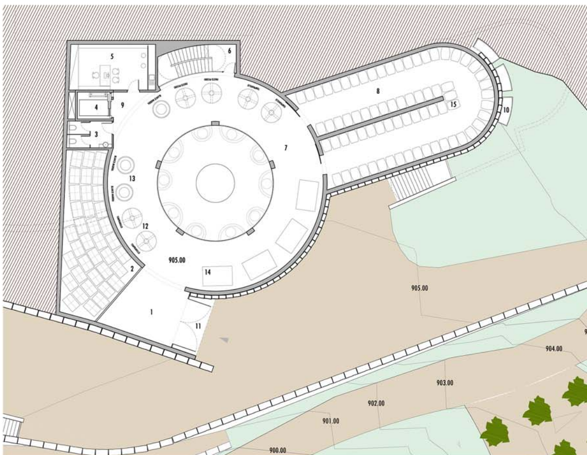
PLANTA -1 E: 1/300
